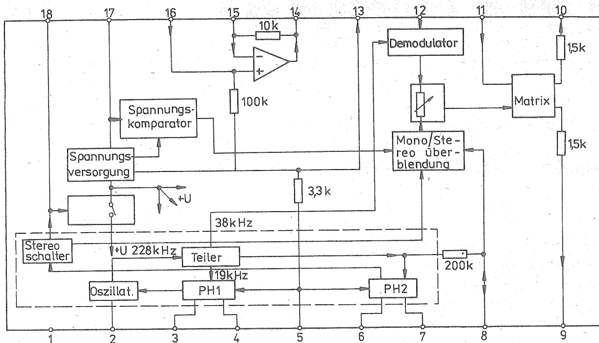
Bild 2: Blockschaltbild
